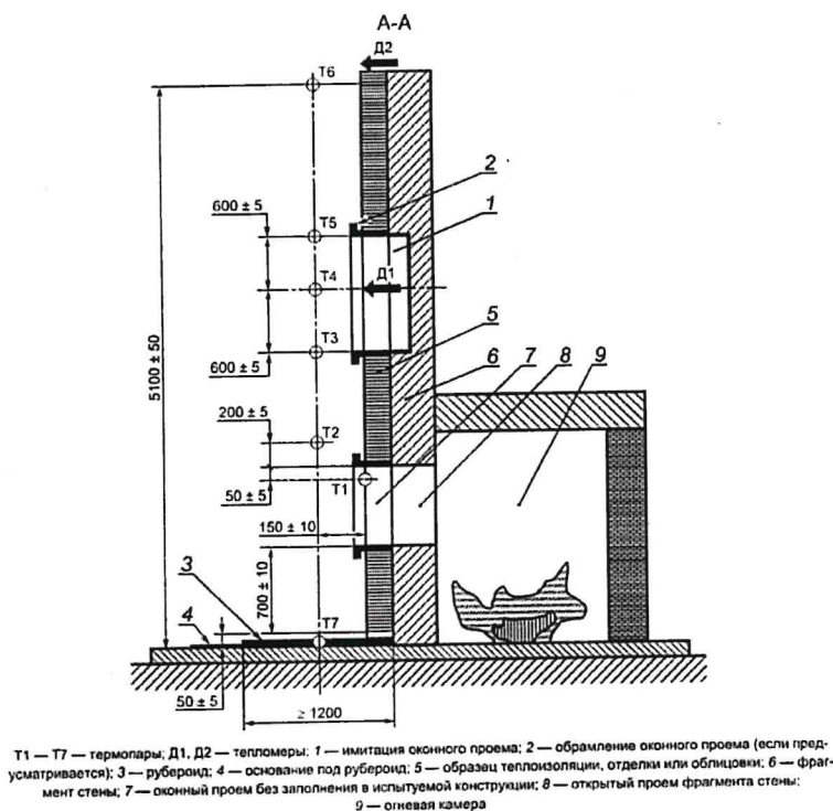
Рис. 3. Схема установки термопар и датчиков теплового потока при испытаниях.
