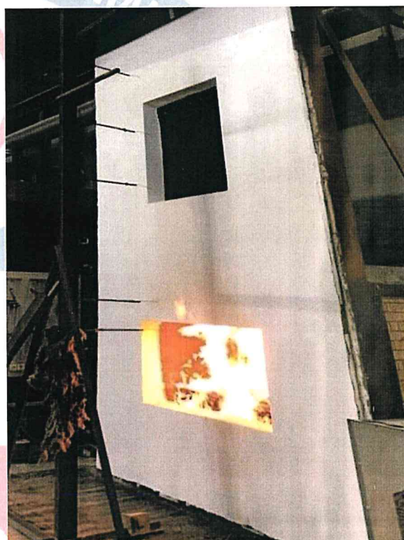
Рисунок 2. Общий вид образца СФТК в начале испытаний.
