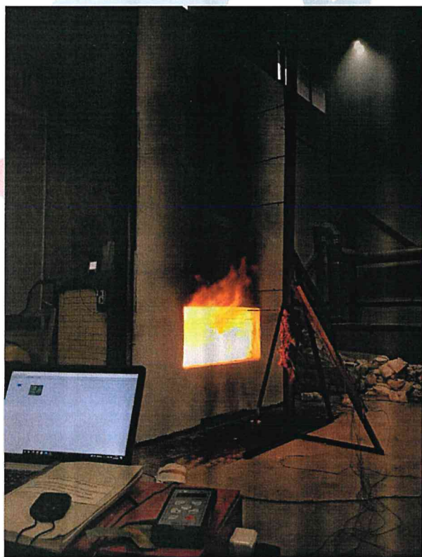
Рис. 8. Внешний вид образца на 35-й минуте испытания.
